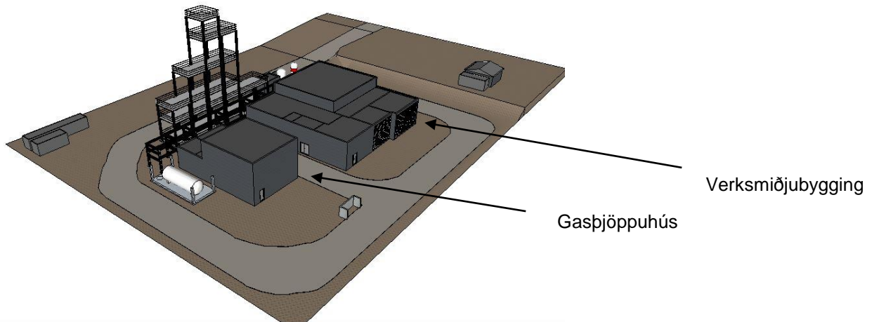
Mynd 7 Verksmiðja eftir stækkun. Sjá einnig mynd 7 og 9.
